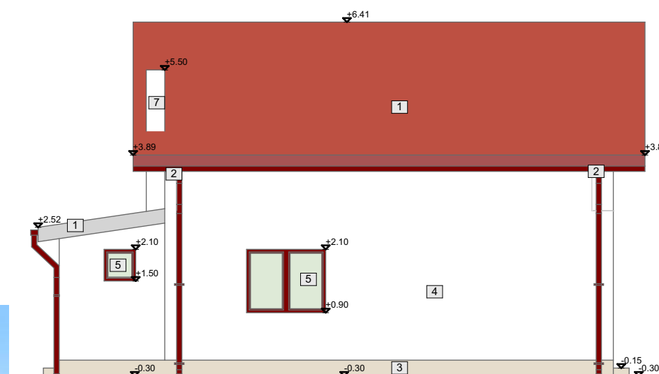
FATADA SUD
